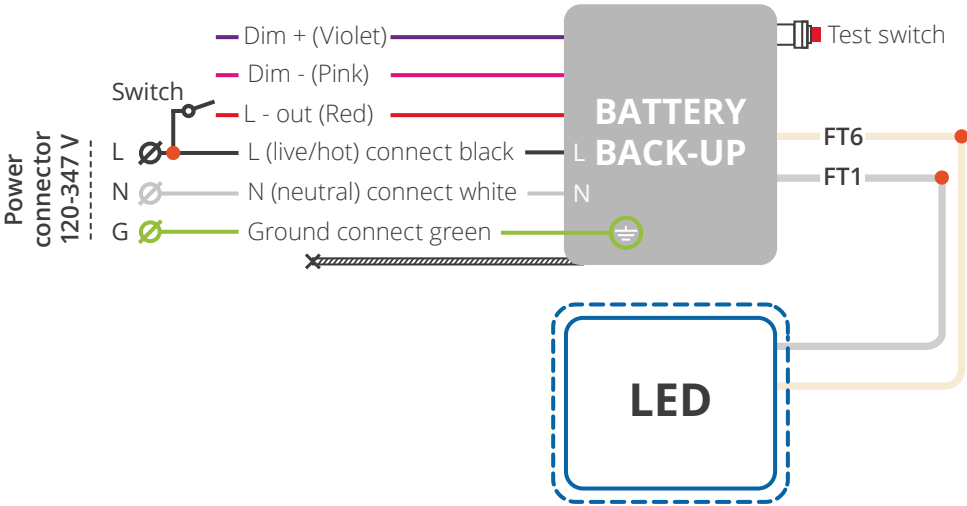
WIRING DIAGRAM (0-10V DIMMABLE/120-347VAC)
